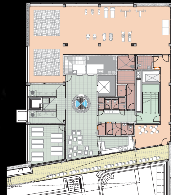
PRVNÍ PATRO
